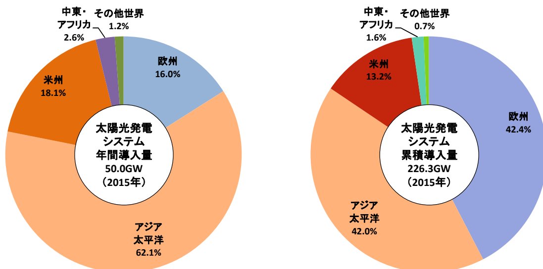
図2 世界における地域別太陽光発電システム2015年導入量および累積導入量内訳
