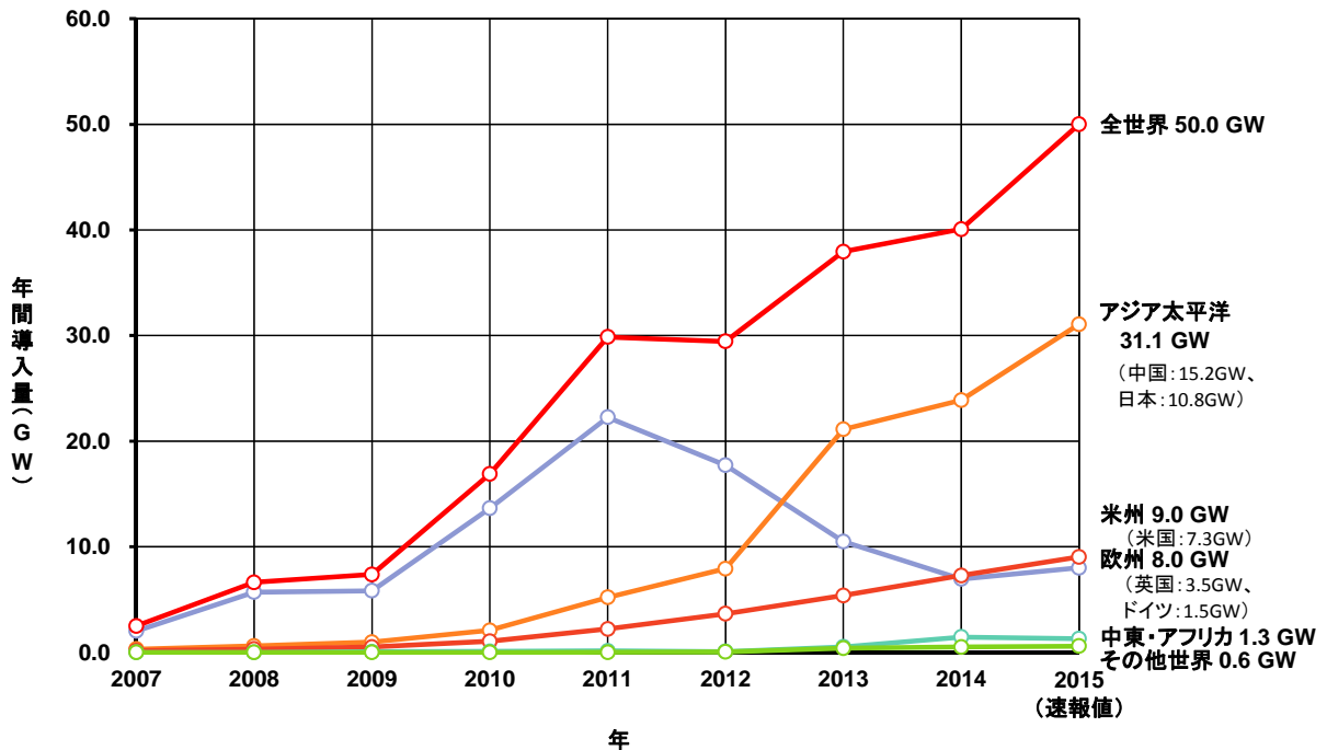
図1 世界における地域別太陽光発電システム年間導入量推移
