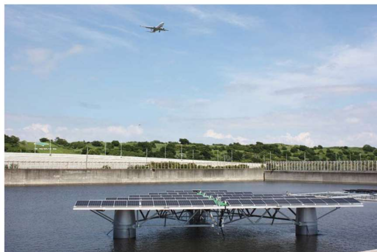
東京都・東京ベイエリア洋上浮体式太陽光発電設備・80～100kW
